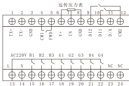
XLP-HK10(S)型控制器端子接线图:
